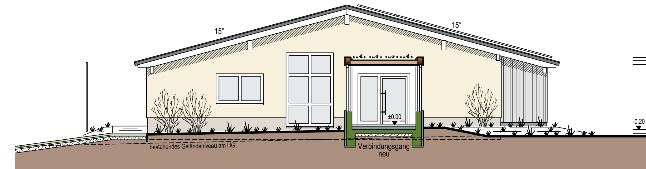
ANSICHT WESTSEITE
