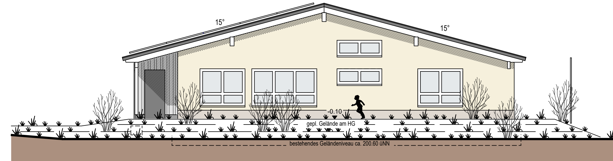
ANSICHT OSTSEITE
